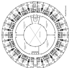
Planta Tipo
