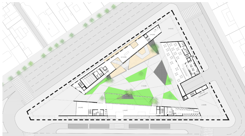
Planta Baja
