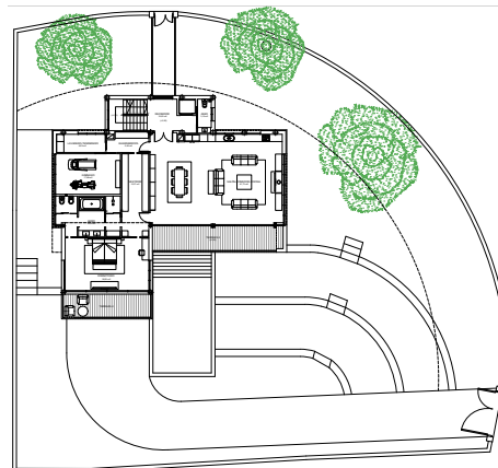
Planta Primera
