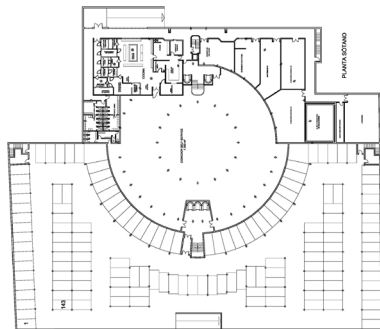
Planta Sótano
